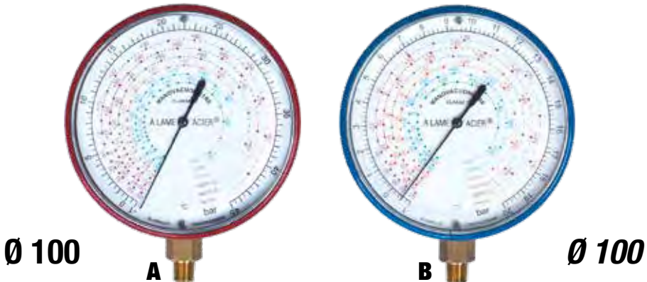
Manometro Blondelle Ø 100 - Att. radiale - Classe 1 Blondelle pressure gauge Ø 100 - Radial - 1 Cl.
